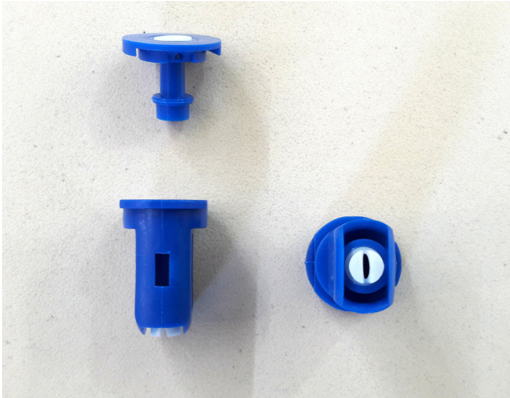
Flachstrahldüse 6 MS 03 C (Keramik, kunststoffummantelt, blau)
